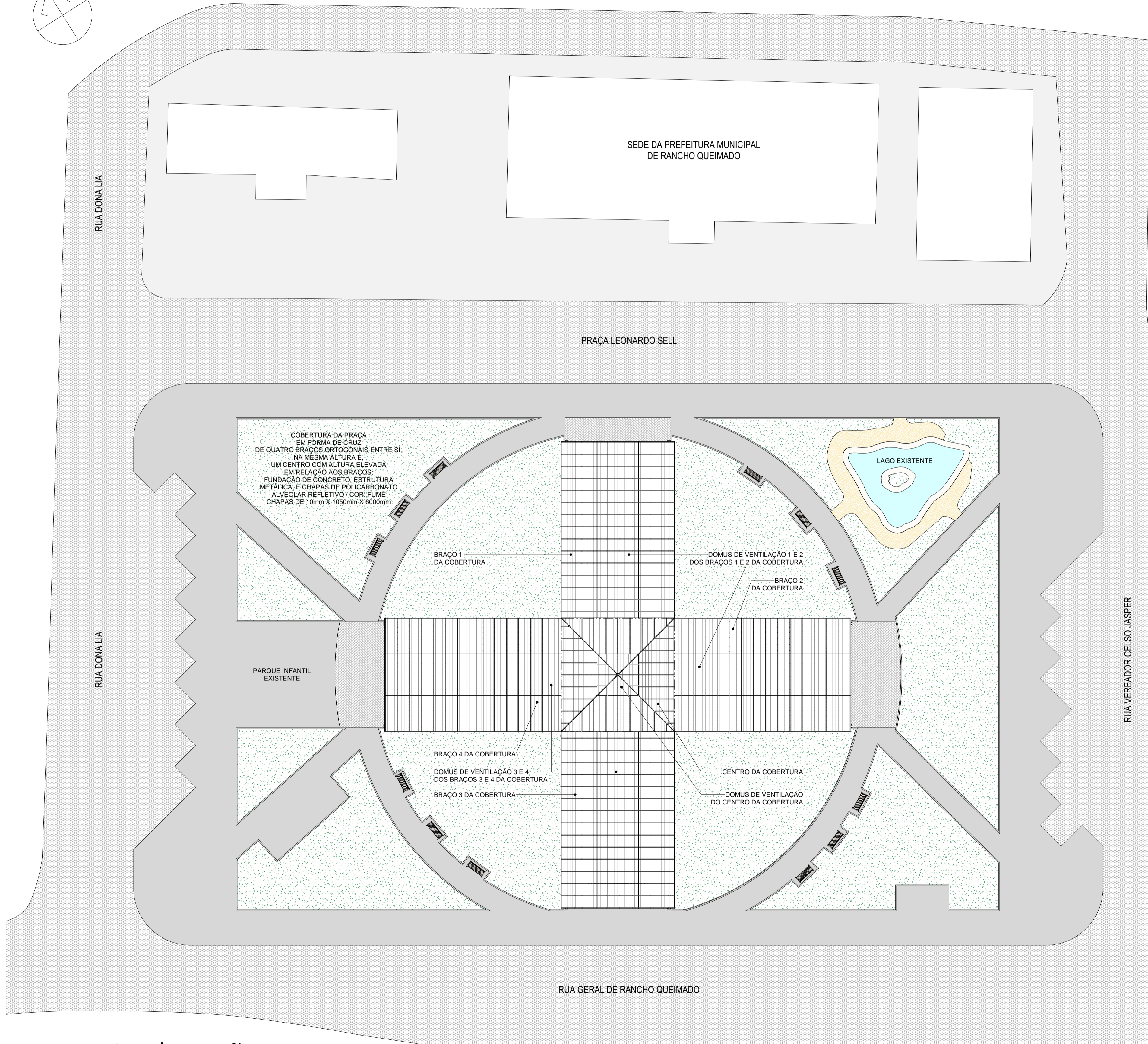
2 Implantação Escala 1 : 200
